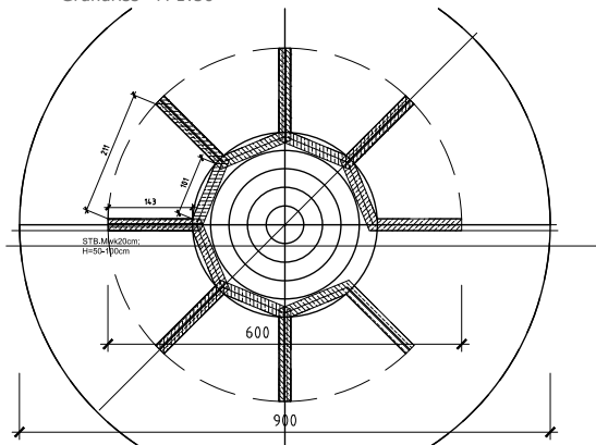
Grundriss M 1:50
